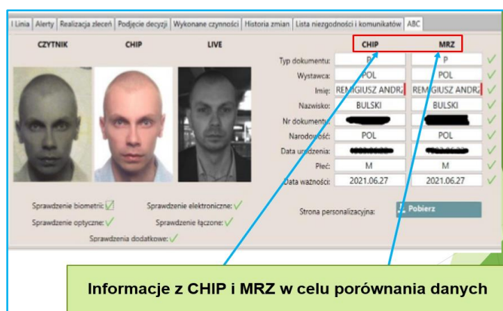
Fot. 19. Sekcja ABC w szczegółach odprawy (porównanie danych z CHIPA i MRZ wizerunku podróżnego) – fot. pochodzi z Podręcznika użytkownika: Zintegrowany System Ewidencji 6
