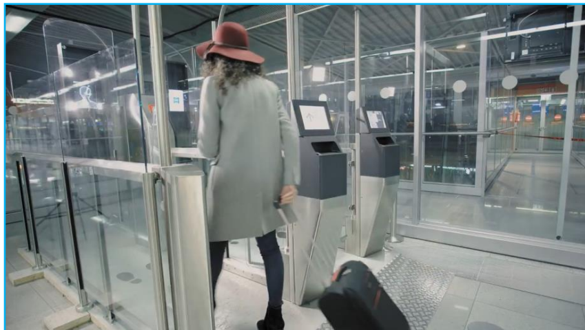
Fot. 26. Otwarcie drzwi wejściowych do bramki ABC po poprawnym odczycie dokumentu
