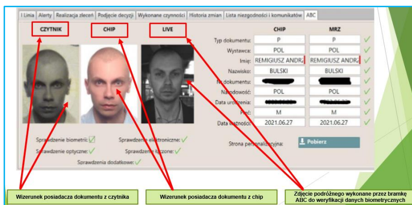
Fot. 17. Sekcja ABC w szczególności odprawy (porównanie wizerunku podróżnego) – fot. pochodzi z Podręcznika użytkownika: Zintegrowany System Ewidencji 6
